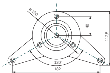
Piastra in alluminio pressofuso attacco ortogonale 90° Alluminium alloy plate for 90° orthogonal connection
