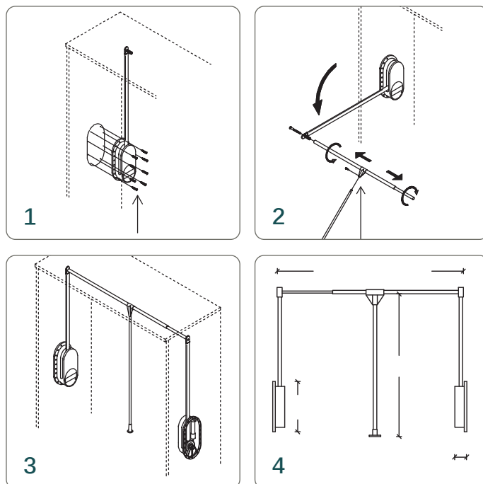
Schema montaggio tipo 1 / Assembly diagram tipe 1
