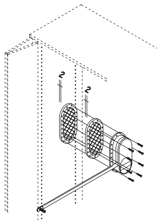
Vista assonometrica Axonometric view
